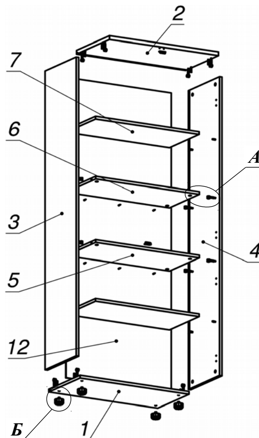
Схема сборки
