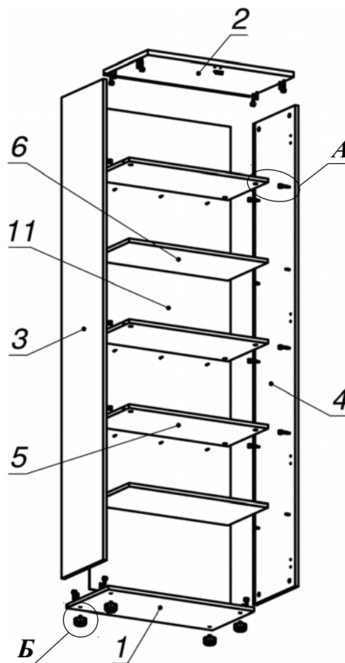
Схема сборки
