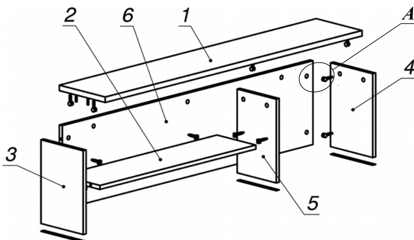
Схема сборки
