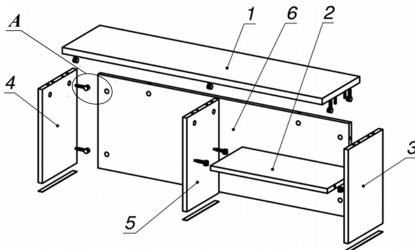
Схема сборки
