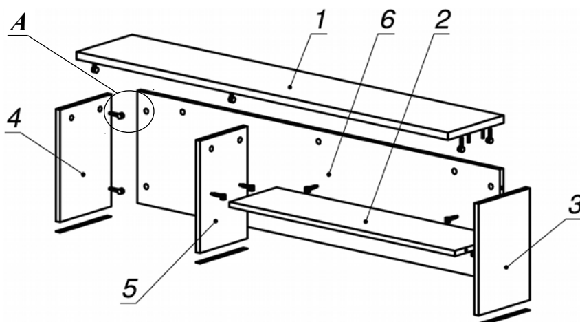
Схема сборки
