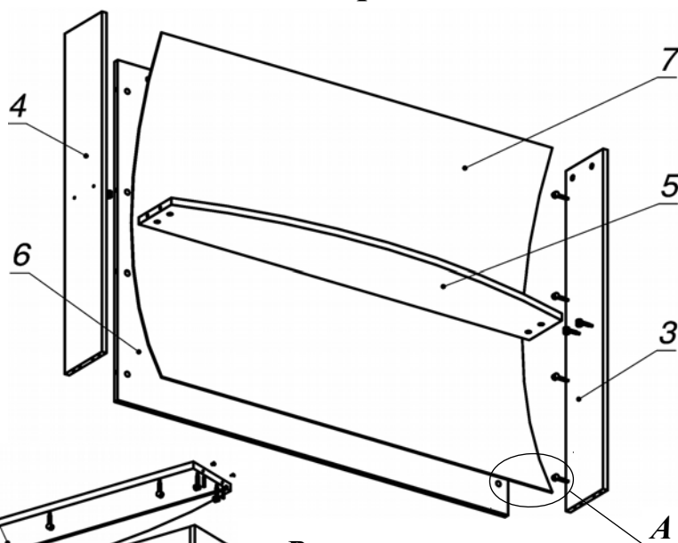
Схема сборки
